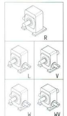
軸向選擇 Shaft Direction 單位: m/m
