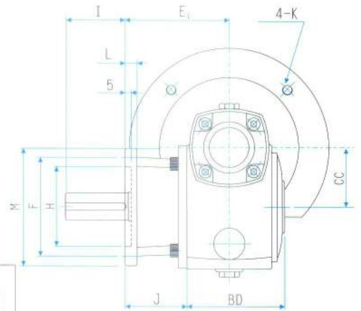
出力軸 Output shaft
